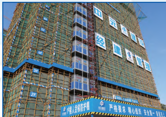
定型化转料平台安全牢固、外立面整洁美观
